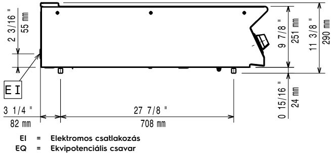
Felülnézet
